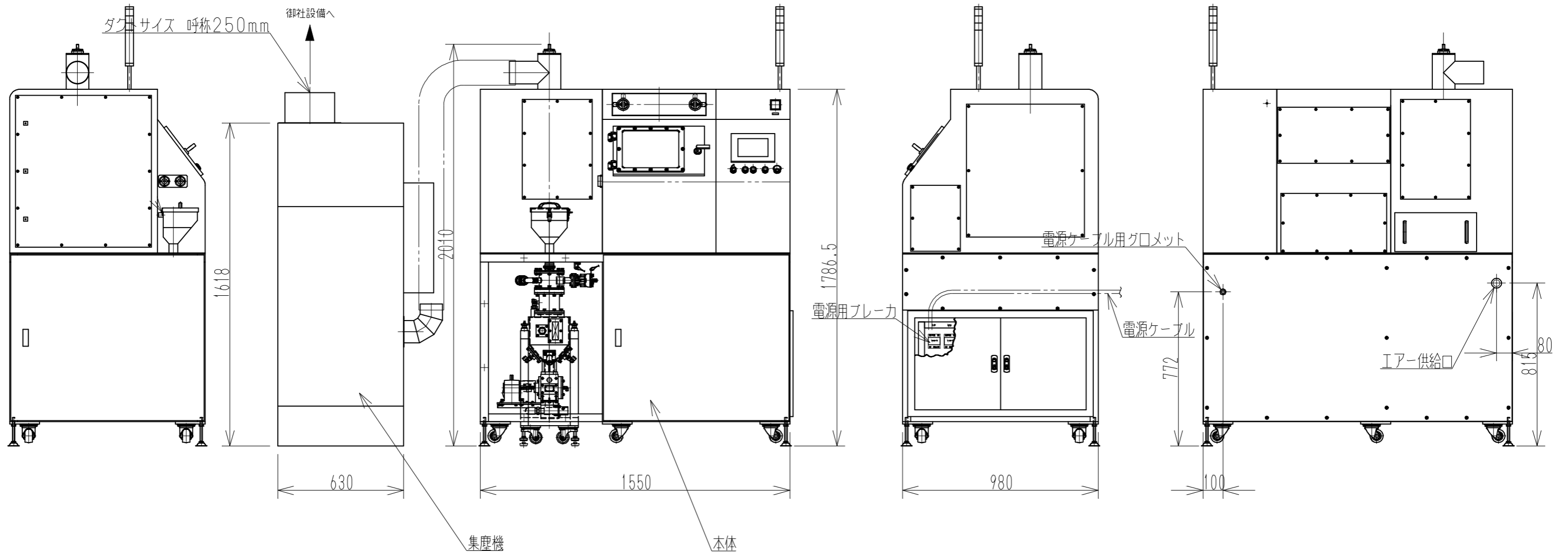
外観図
